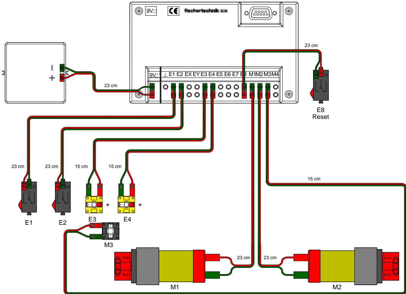
Elektrischer Schaltplan Circuit diagram Plan électrique
